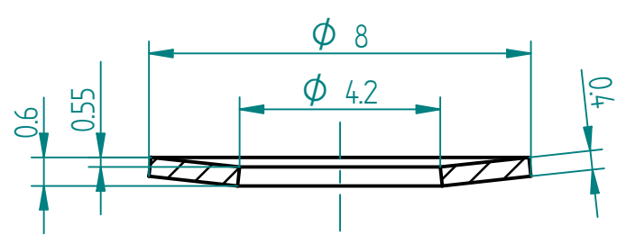
剖面 A-A
