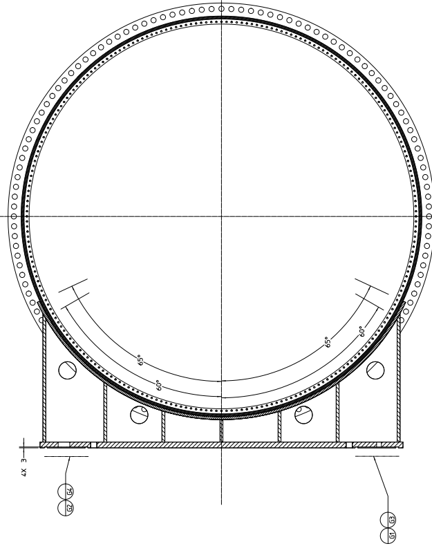
Section D-D
