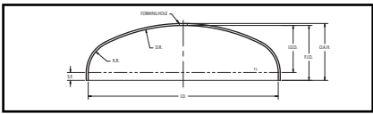
2:1 Elliptical
