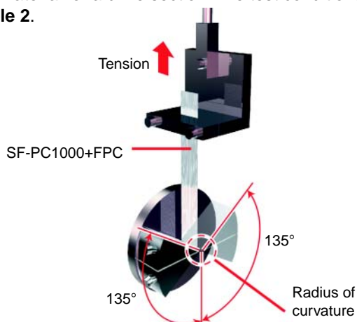
Fig. 4 MIT flexural endurance test
