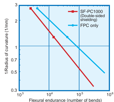
Fig. 5 MIT flexural endurance characteristics
