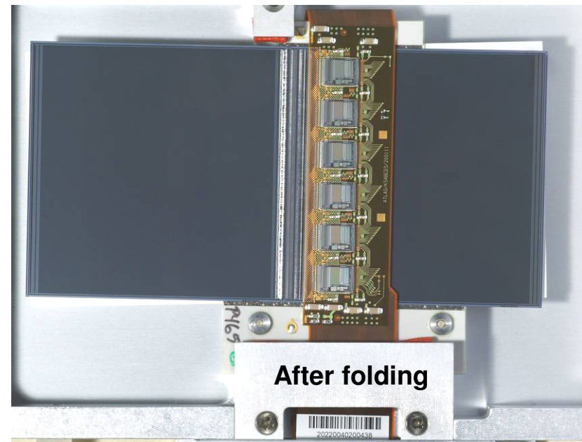
Atlas SCT module
