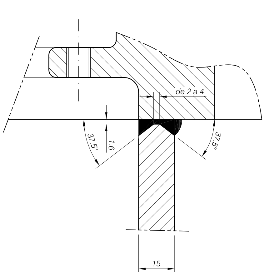
SOLDADURA FONDO-BRIDA
