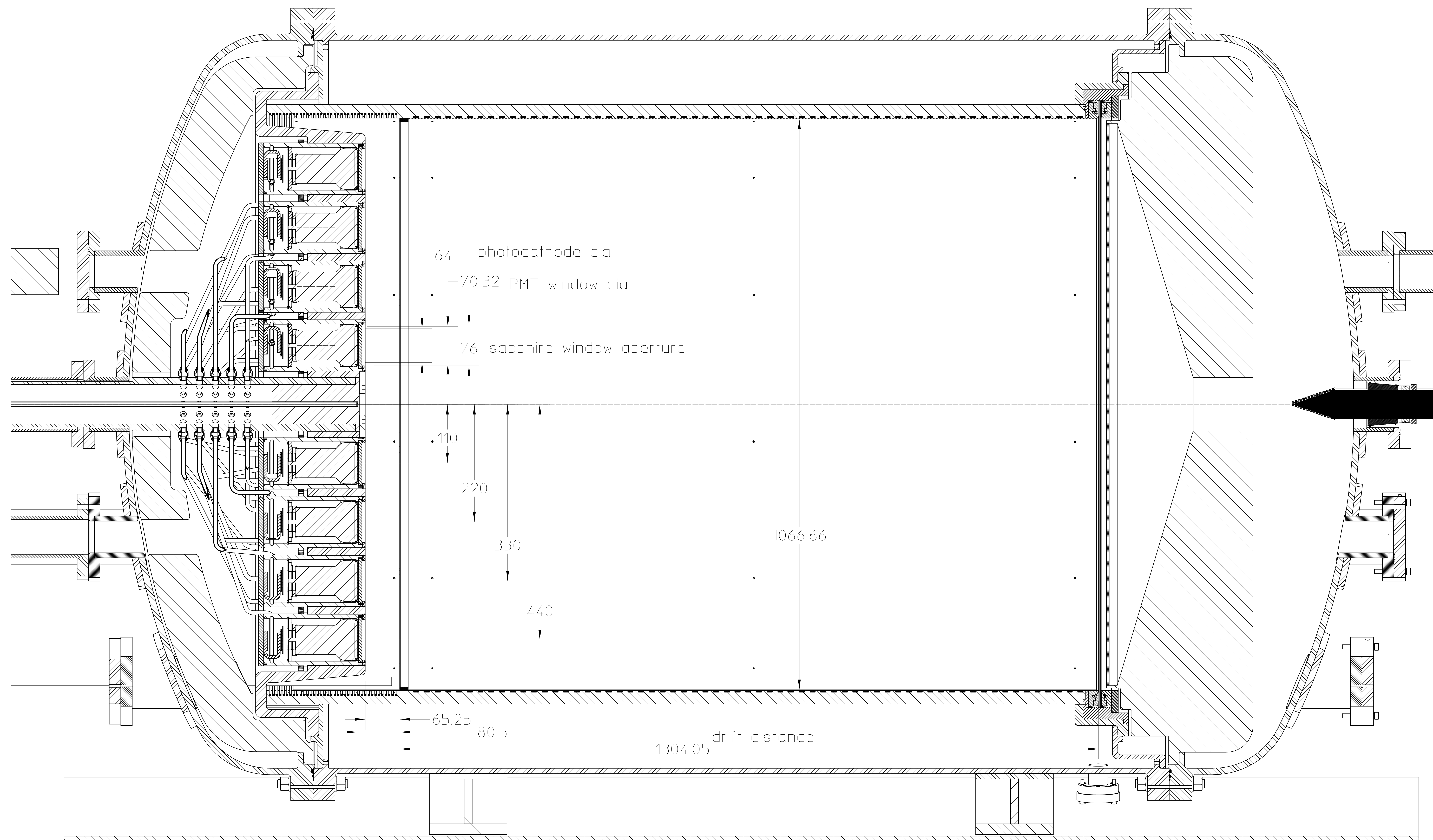
Section D-D
