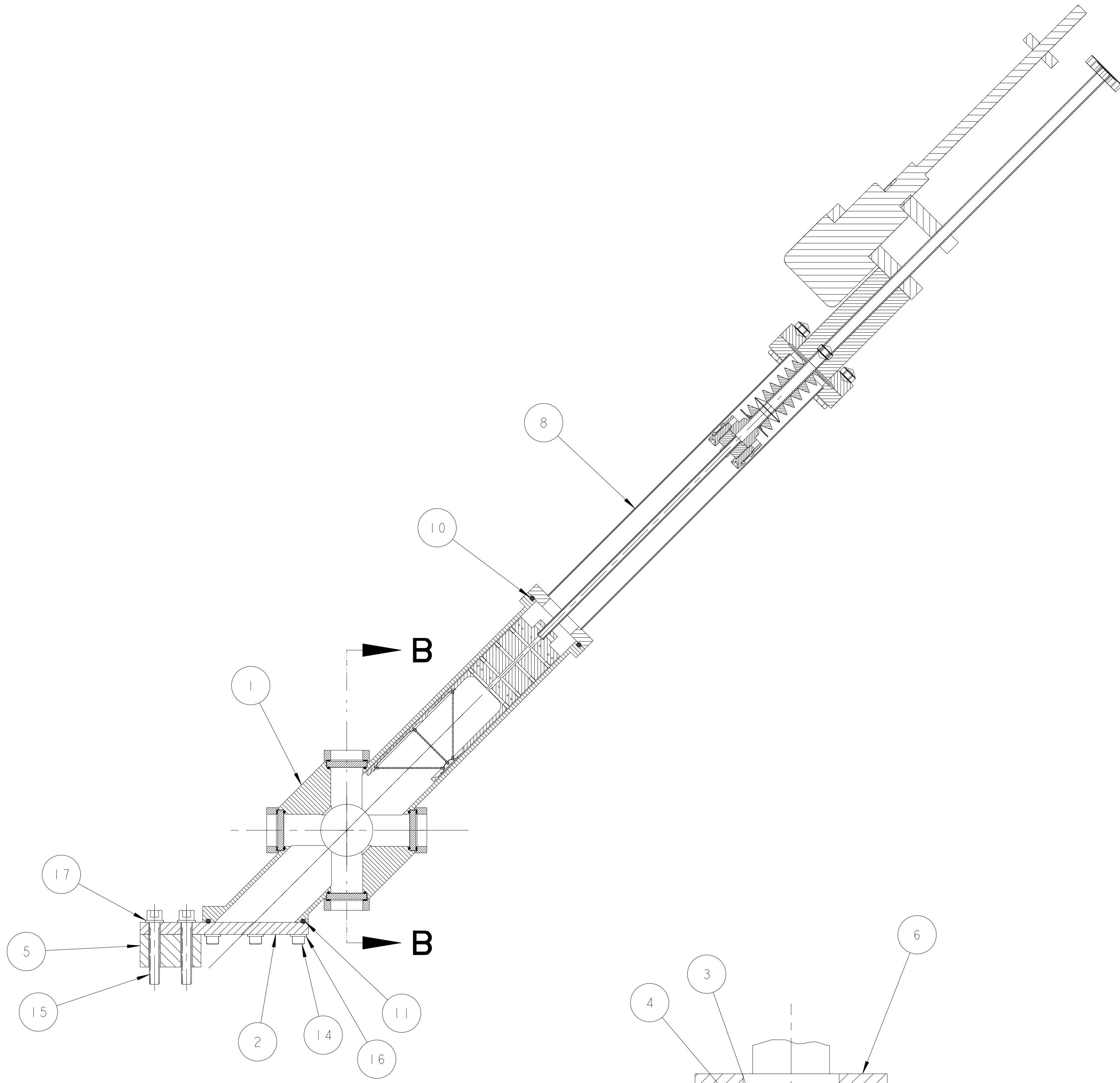
SECTION A-A
