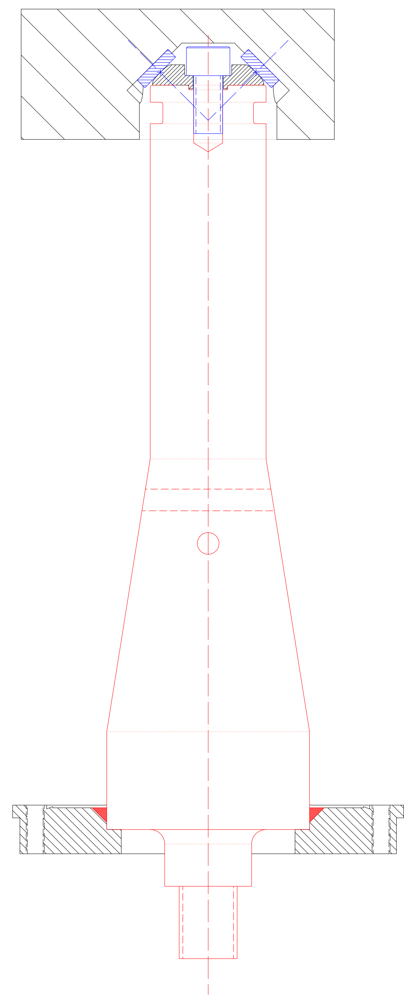
SECTION A-A
