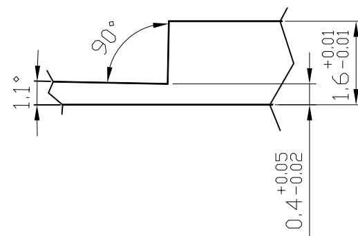
Detail 1 (10:1)
