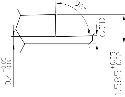
Detail 1 (10:1)
