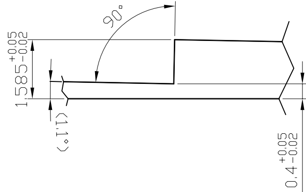
Detail 2 (10:1)
