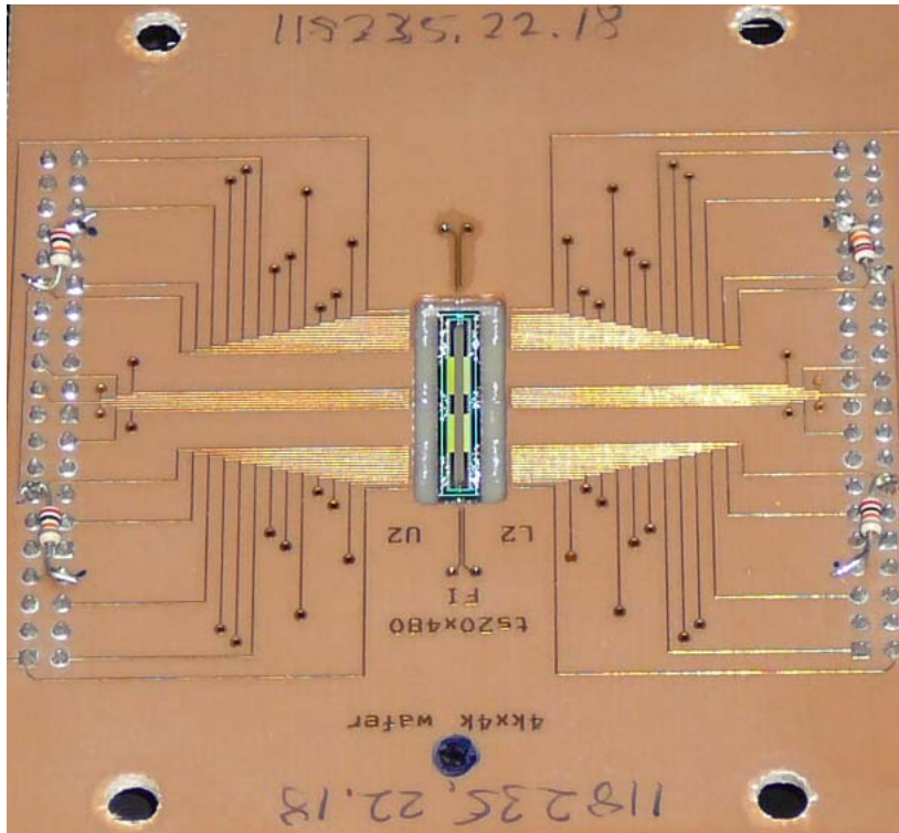
20 x 480 FRONT-ILLUMINATED CCD
